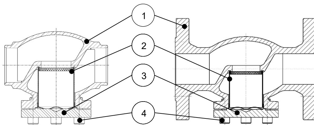
DN10 - 150
