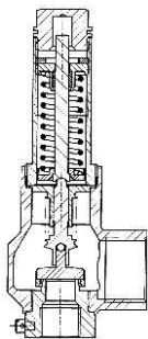
Art.-Nr. 06800 (Muffe) Art.-Nr. 06801 (Zapfen)
